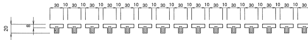
A-A断面図
