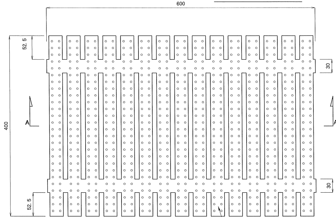
平面図
