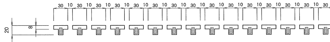
A-A断面図
