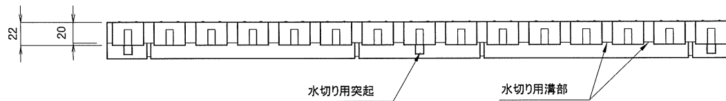
側面図
