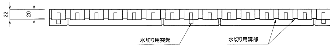
側面図
